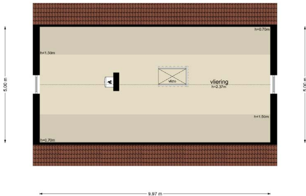
Eerste verdieping
